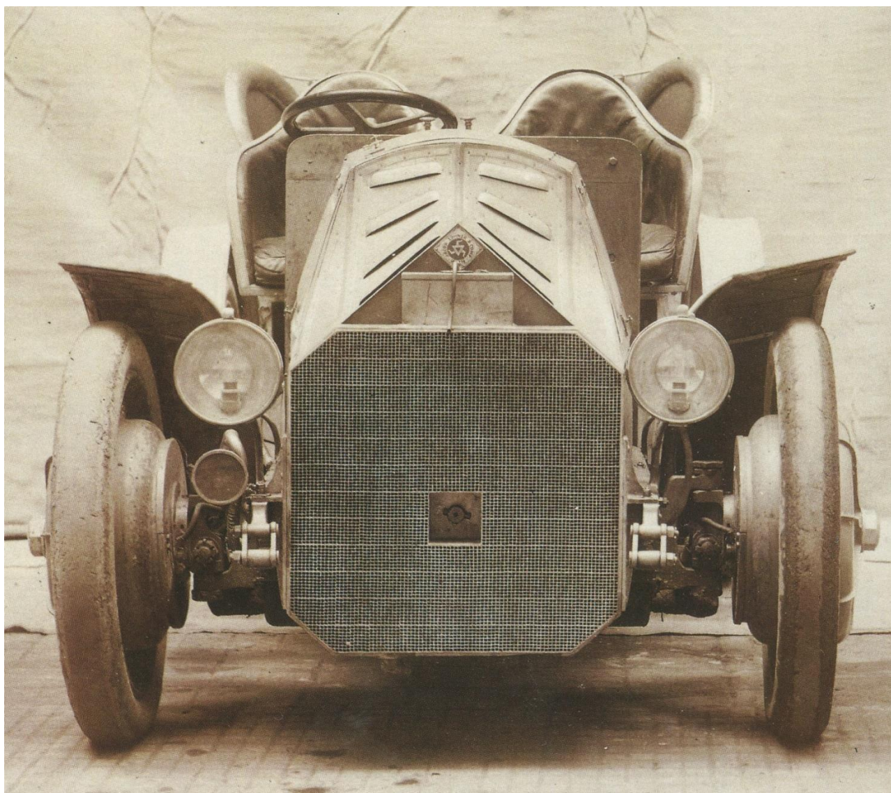
Lohner-Porsche Type Mixte 1902 Benzingenerator – Elektro Radnaben Motoren
